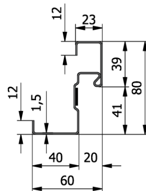
Detalle Marco
