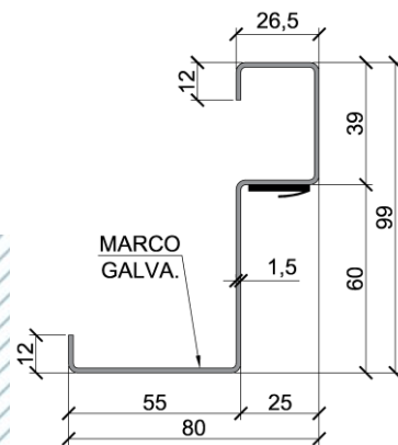
Detalle marco
