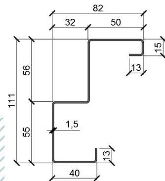
Detalle marco
